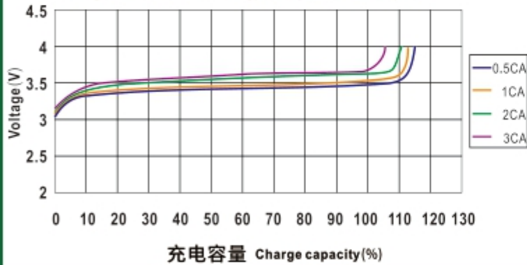
常温下LYP类电池的充电特性曲线
